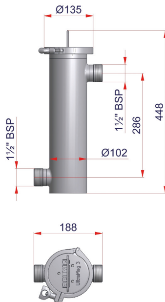
Puhdistusasema 1, 3 ja 3-600 Ultra Mag-malleille
