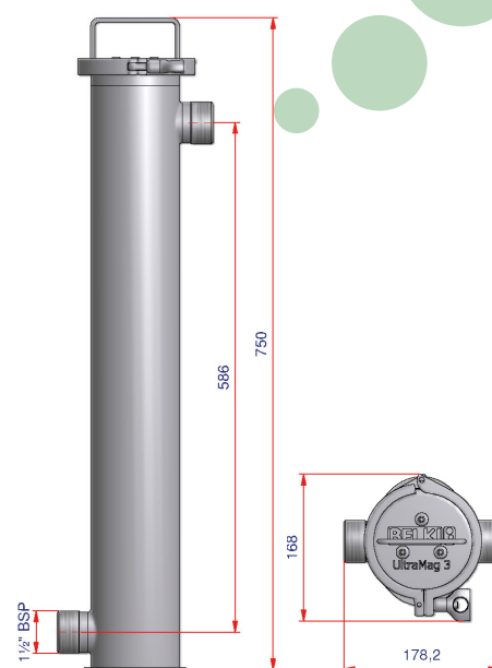
Puhdistusasema 1, 3 ja 3-600 Ultra Mag-malleille
